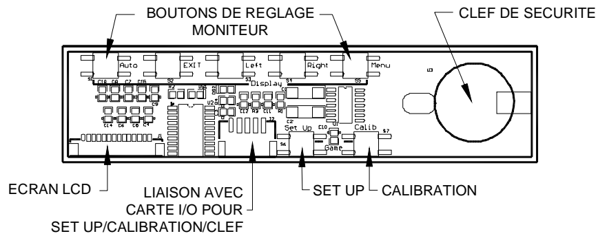
ILLUSTRATION 50 - DESSIN CARTE REGLAGE MONITEUR
