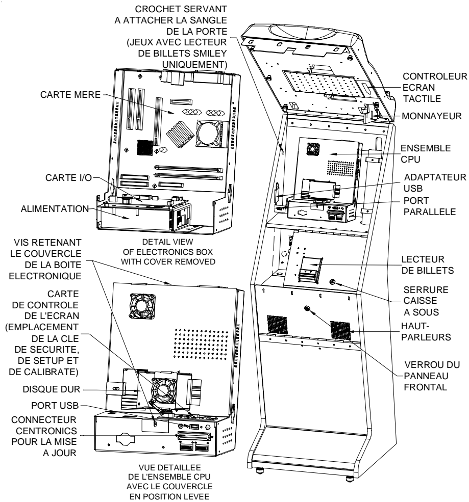
ILLUSTRATION 45 - VUE AVANT FUSION AVEC ENTOURAGE D'ECRAN SOULEVE
