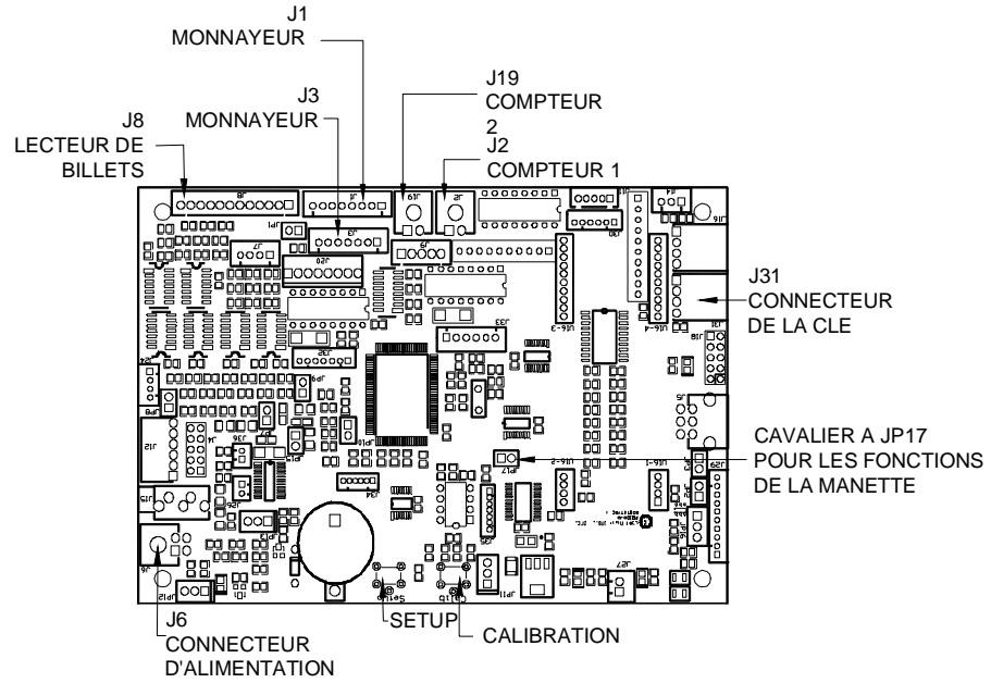
ILLUSTRATION 49 - DESSIN CARTE I/O
