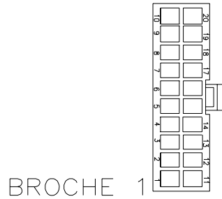
ILLUSTRATION 48 - CONNECTEUR - VUE ARRIERE
