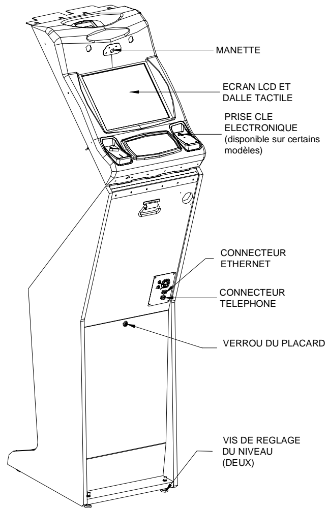
ILLUSTRATION 46 - VUE ARRIERE FUSION AVEC ENTOURAGE D'ECRAN SOULEVE
